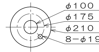
吸込・吐出フランジ寸法
