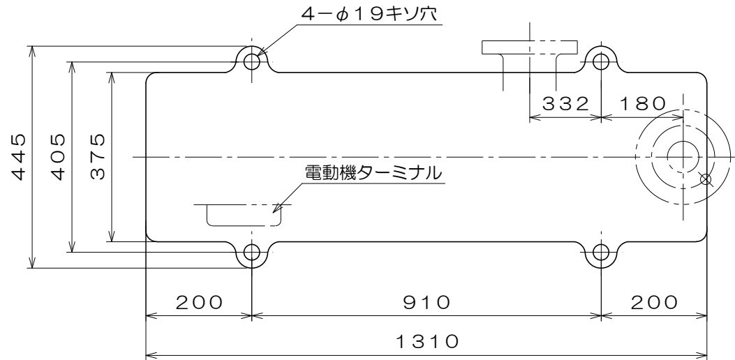
A視図
