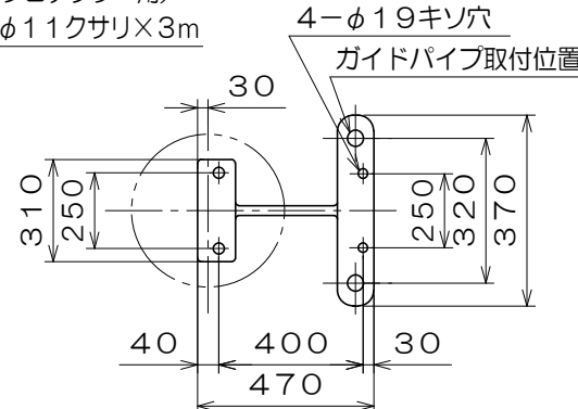
基礎部寸法
