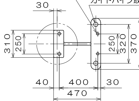
基礎部寸法
