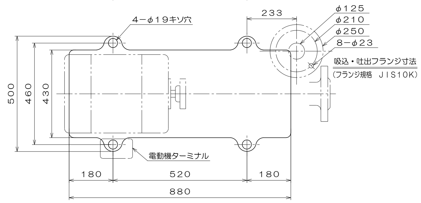
A 視図
