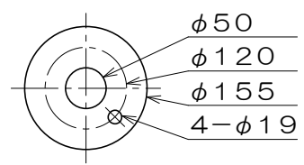
吸込・吐出フランジ寸法
