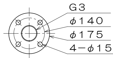
相フランジ寸法
