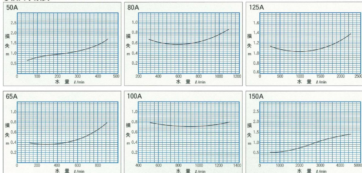
●損失水頭表
